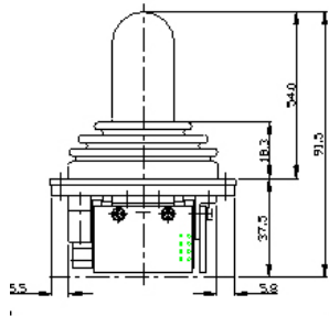
Dimensions MJ-3K CP 54
